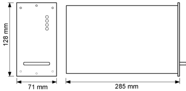
Figure 8.) Module dimensions
