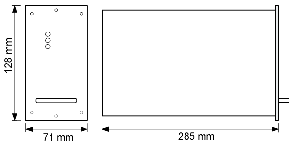
Figure 7.) Module dimensions
