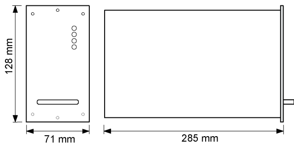
Figure 7.) Module dimensions
